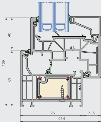
Secțiune verticală
