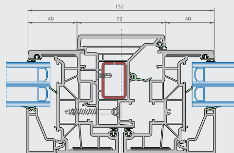
Secțiune orizontală
