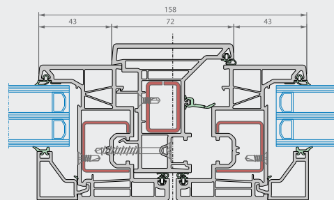
Secțiune orizontală
