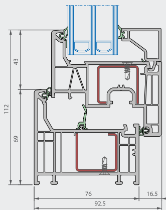
Secțiune verticală
