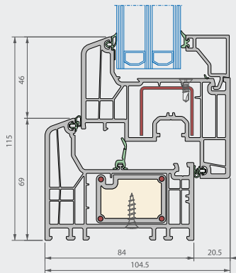
Secțiune verticală
