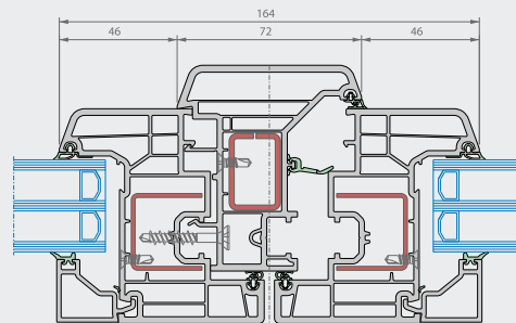
Secțiune orizontală
