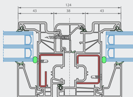
Secțiune orizontală
